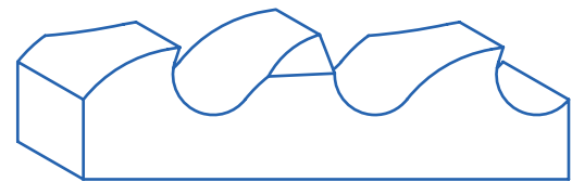
BW - DIENTE CURVO CON CHAFLANES ALTERNADOS
